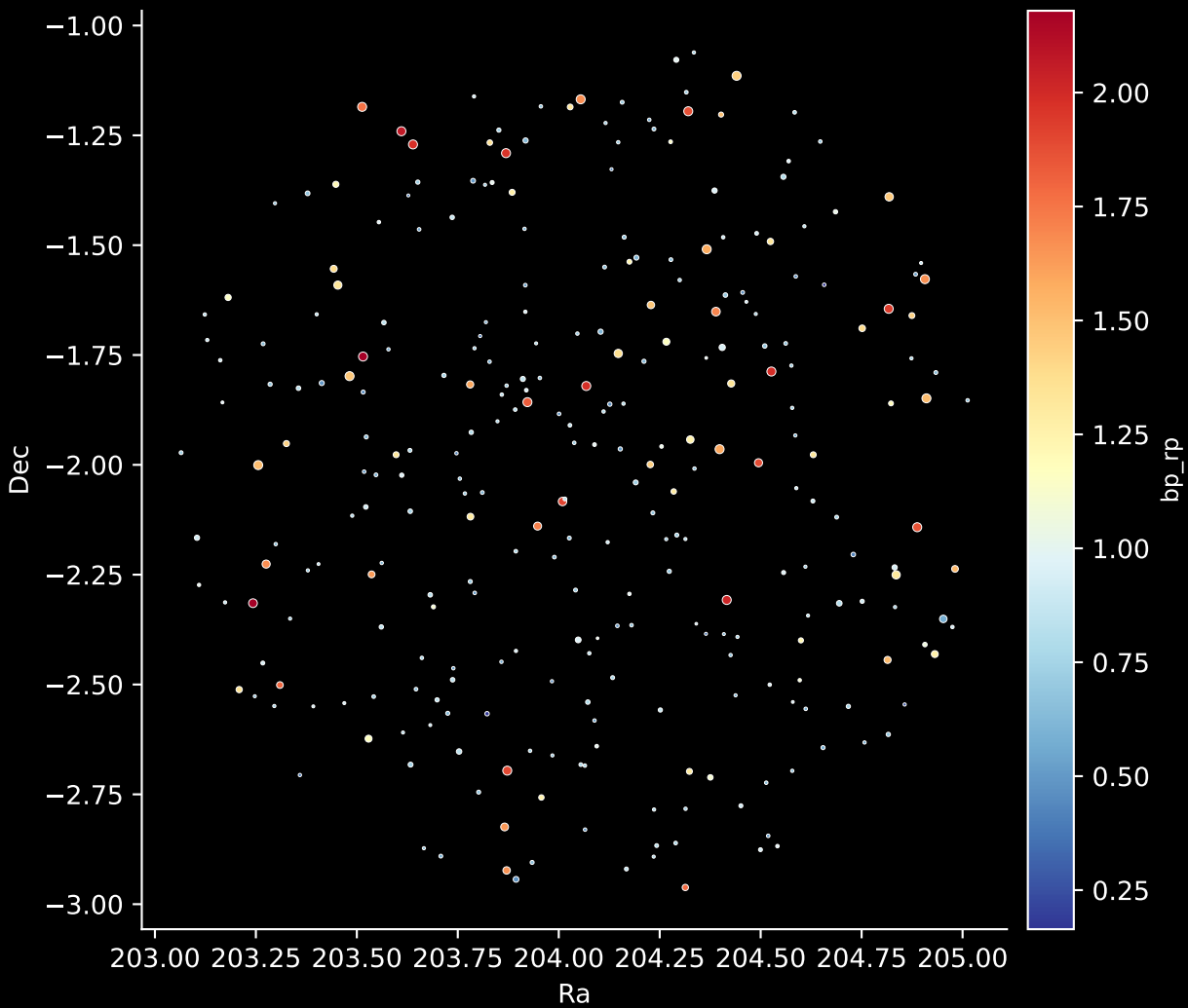
GALAH DR4 Field: [9161] Stars: 287
