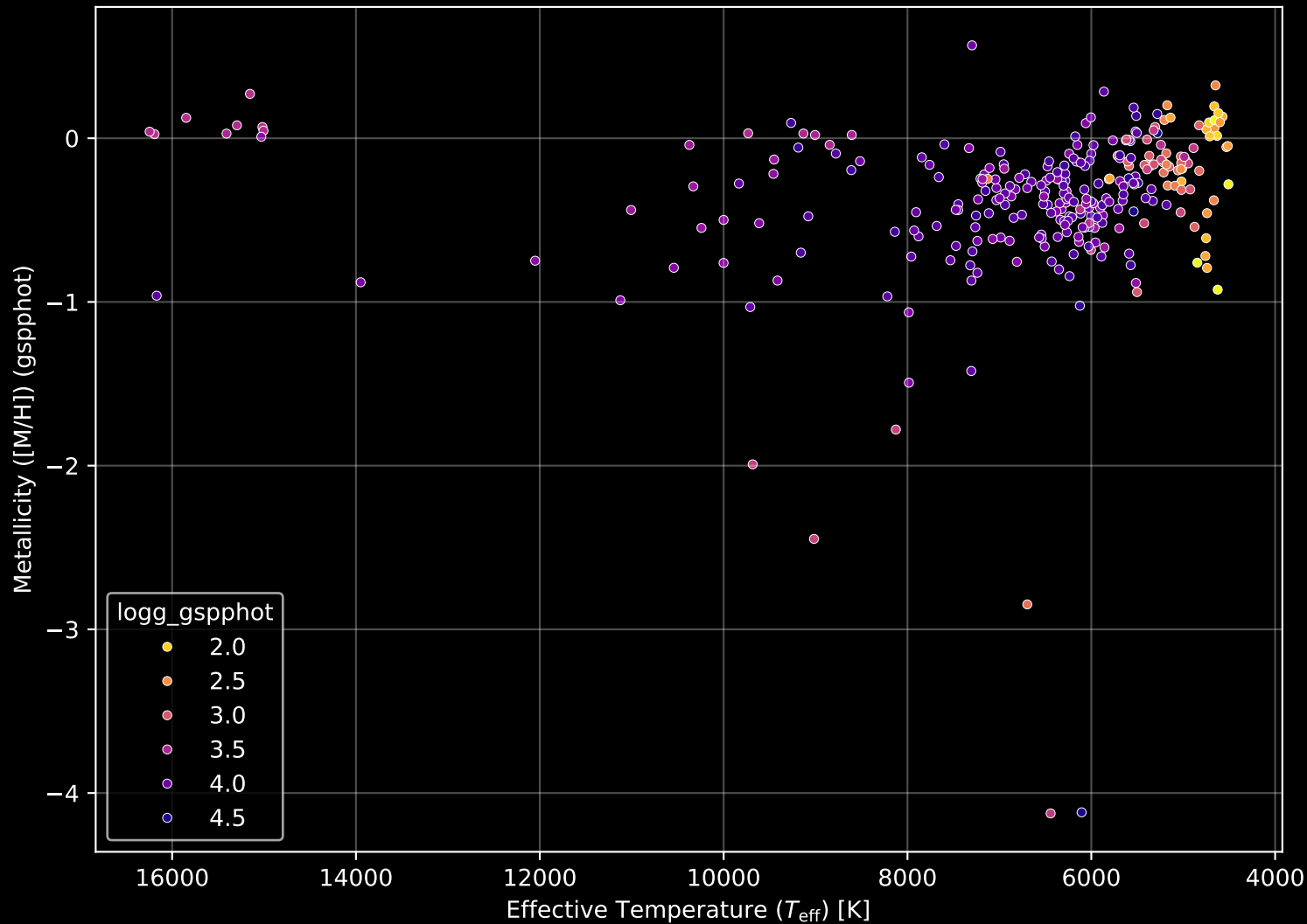
GALAH DR4 Field: [9161] Stellar Population Parameters (n= 287)
